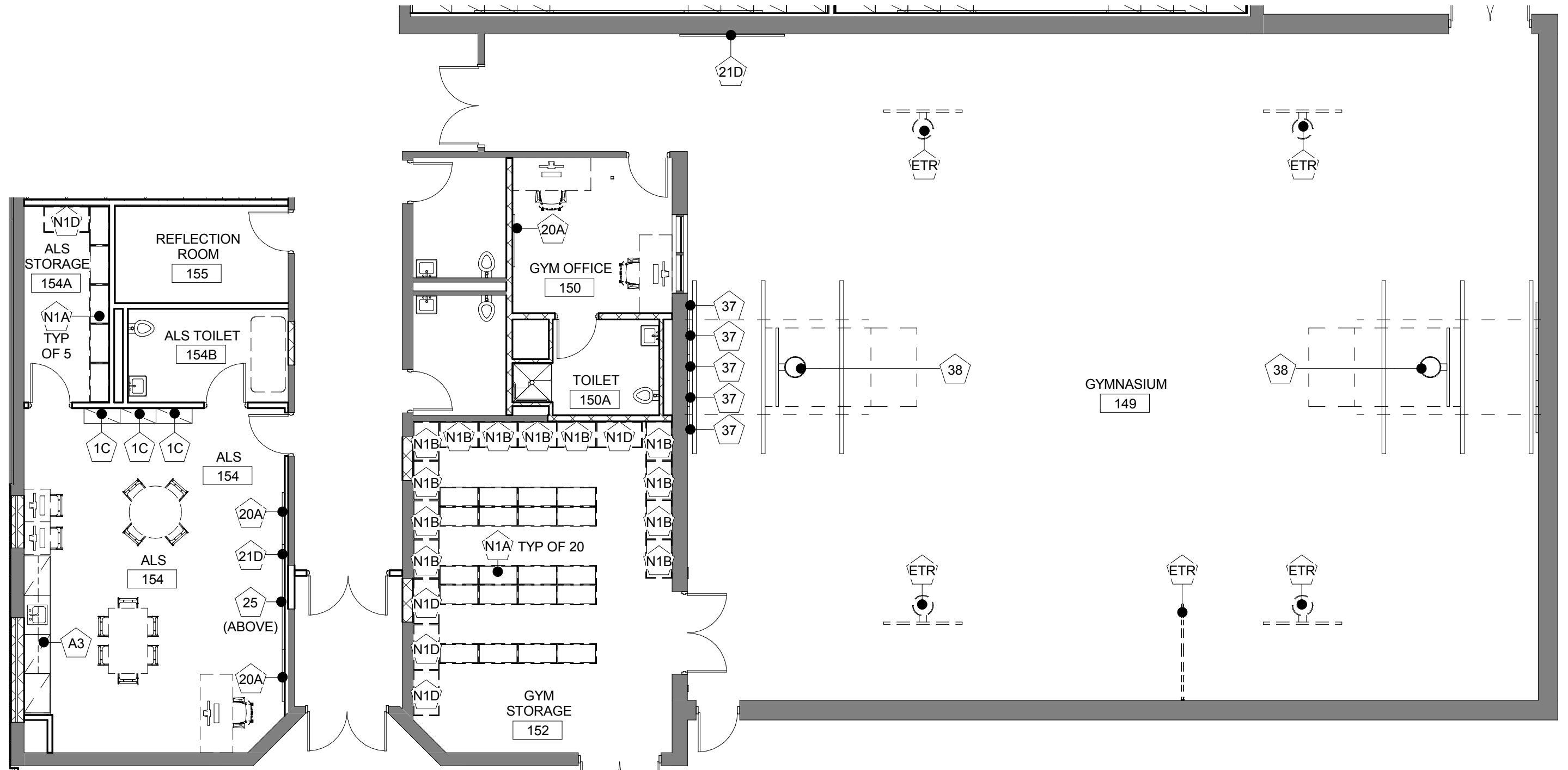
1 GYMNASIUM/ ALS 1/8" = 1'-0"
